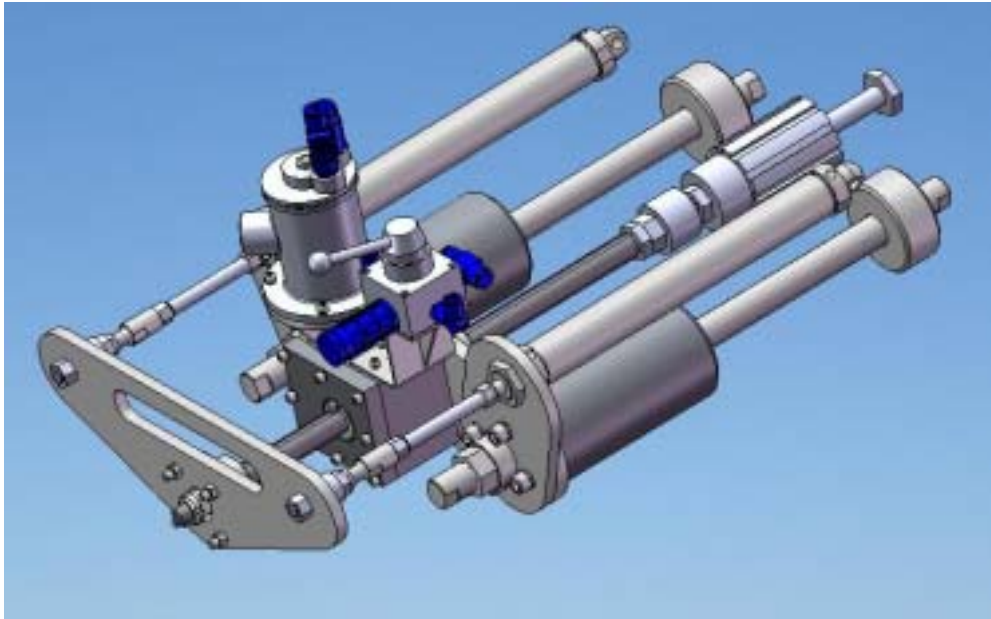
现场磨孔机
